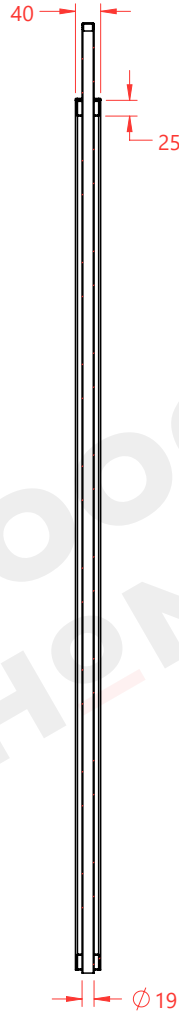
SECTION A-A
